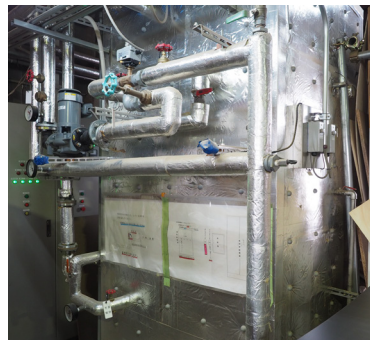
工場から出る廃材を利用した暖房システム
